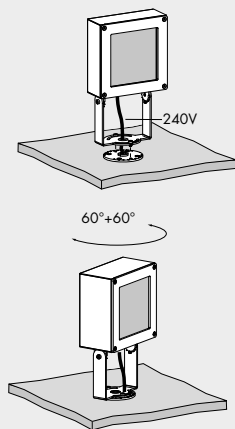
flangia per rotazione 120° f9.009.01 rotation flange
